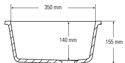
Dwarsdoorsnede zijaanzicht
