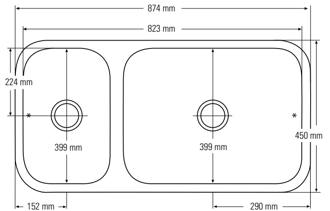
Bovenaanzicht * Overloop
