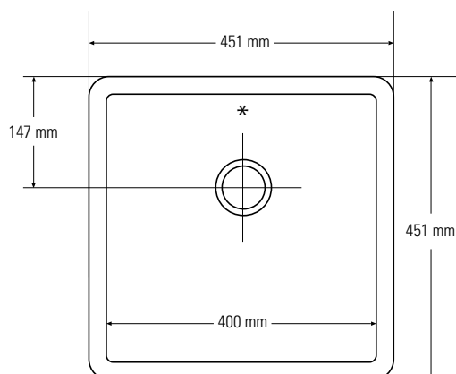
Bovenaanzicht * Overloop
