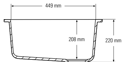
Dwarsdoorsnede zijaanzicht
