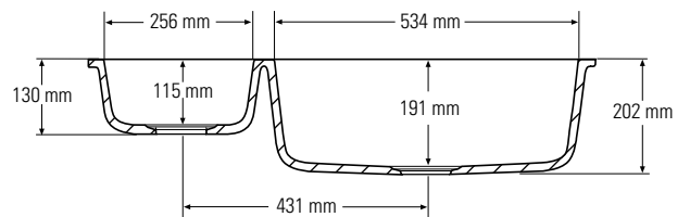
Dwarsdoorsnede frontaal
