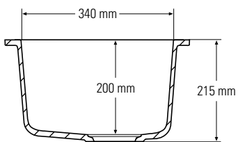
Dwarsdoorsnede zijaanzicht
