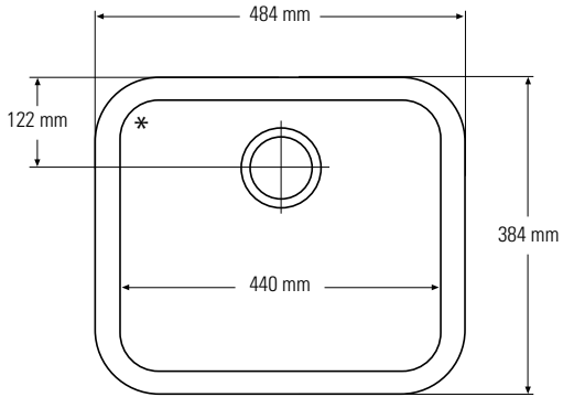
Bovenaanzicht * Overloop
