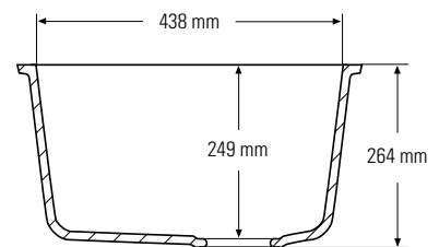
Dwarsdoorsnede zijaanzicht
