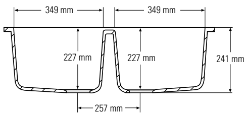
Dwarsdoorsnede frontaal
