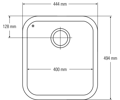
Bovenaanzicht * Overloop
