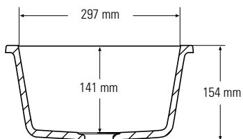
Dwarsdoorsnede zijaanzicht
