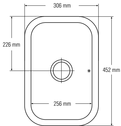
Bovenaanzicht * Overloop
