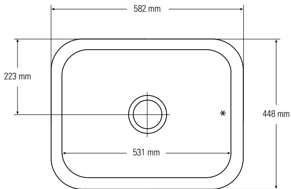
Bovenaanzicht * Overloop
