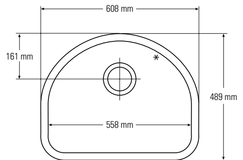
Bovenaanzicht * Overloop
