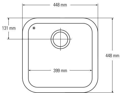
Bovenaanzicht * Overloop
