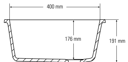
Dwarsdoorsnede zij aanzicht
