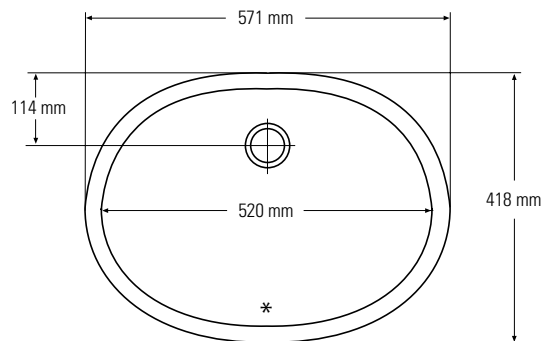
Bovenaanzicht * Overloop
