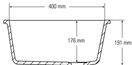
Dwarsdoorsnede zijaanzicht
