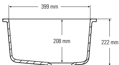
Dwarsdoorsnede zijaanzicht
