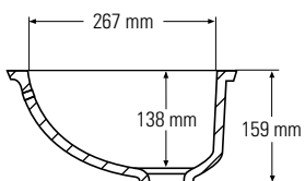
Dwarsdoorsnede zijaanzicht
