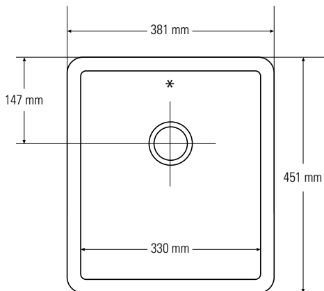
Bovenaanzicht * Overloop
